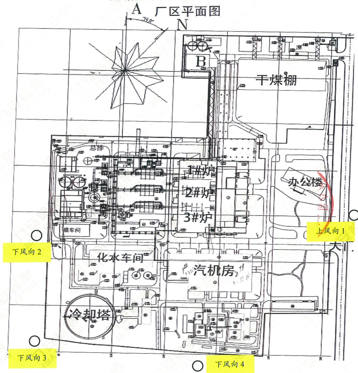
○——无组织废气监测点位 图 1 无组织废气监测点位图
